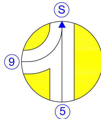
Regard P59 Passage droit + Angle 90° gauche
