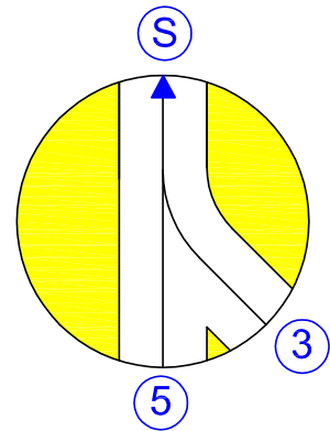
Regard P35 Angle 135° droite + Passage droit
