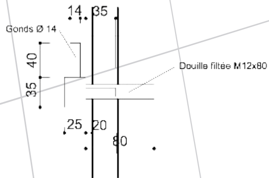
Dimensions précadre EURO-BAIE
